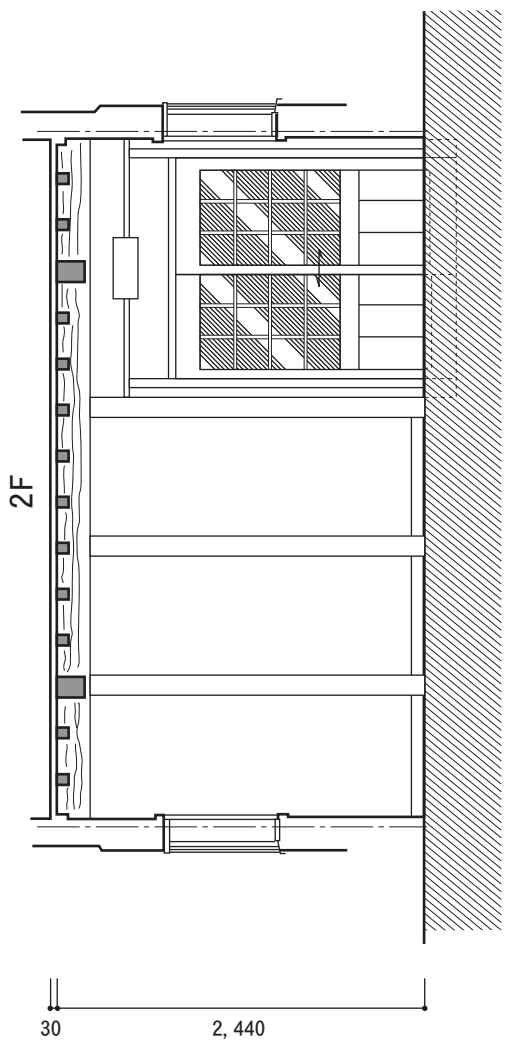
西側立面
